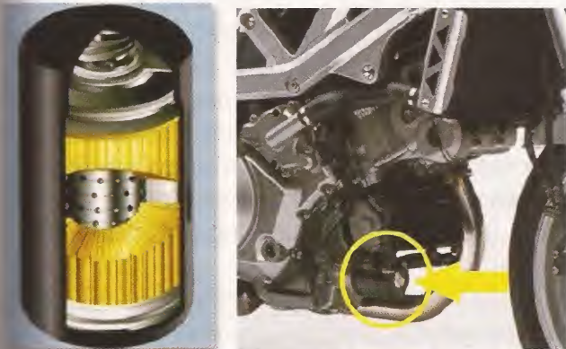
Corte y ubicación del filtro de aceite
